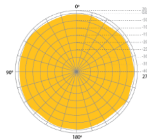
5GHz 2D 無線場形 @ 水平方向
